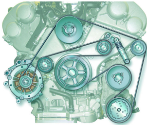
Componentes de la transmisión por correa
