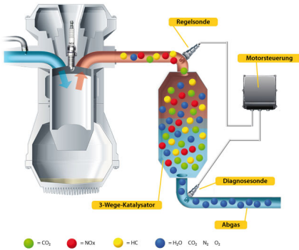
Circuito de control Lambda
